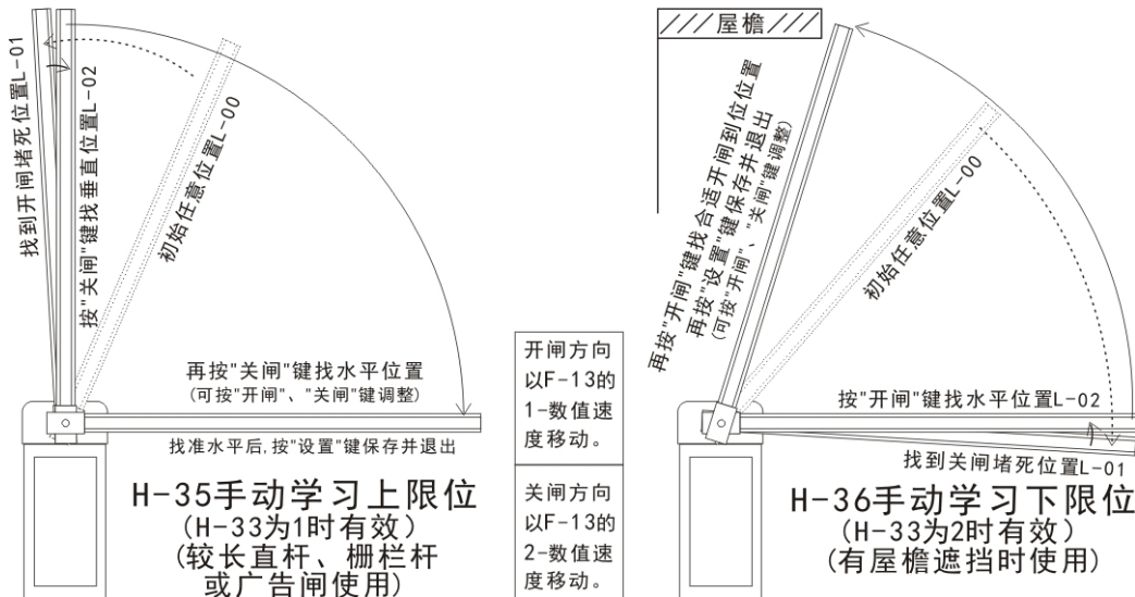
图5-5 H-35 和 H-36 图示
