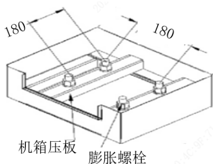
图3-1 打孔间距
