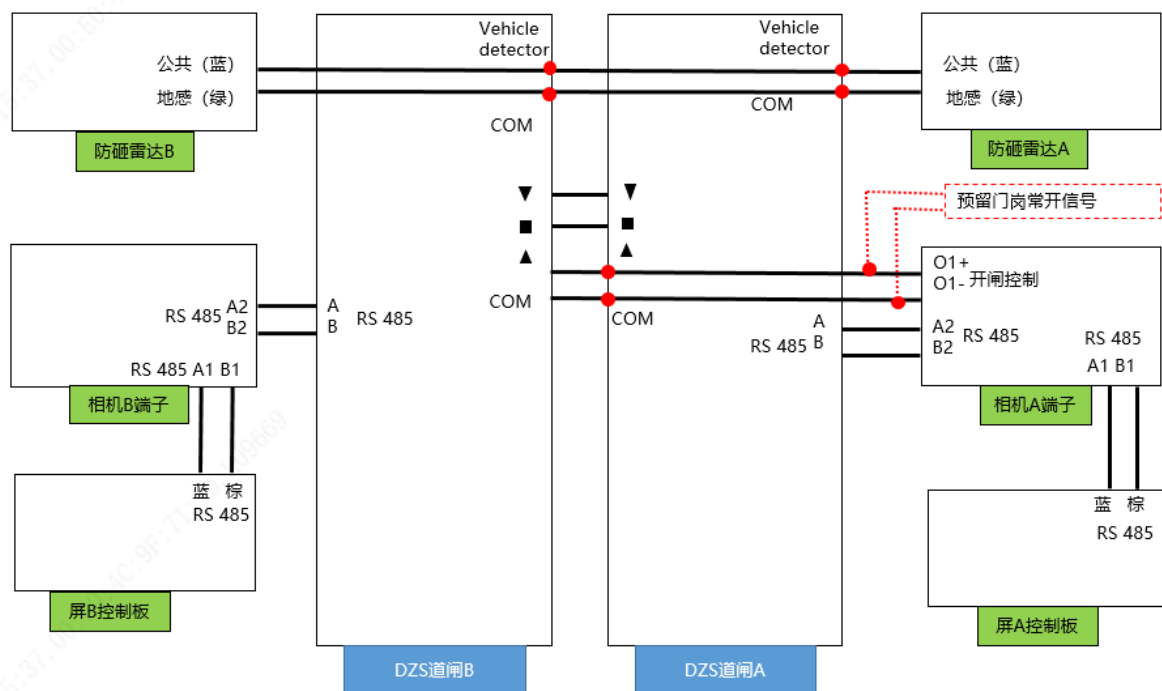
图4-7 道闸对开接线图
