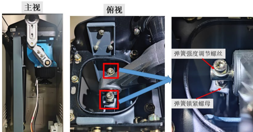
图3-19 机芯结构图
