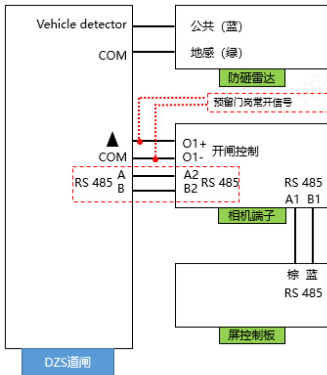
图4-2 整体接线示意图
