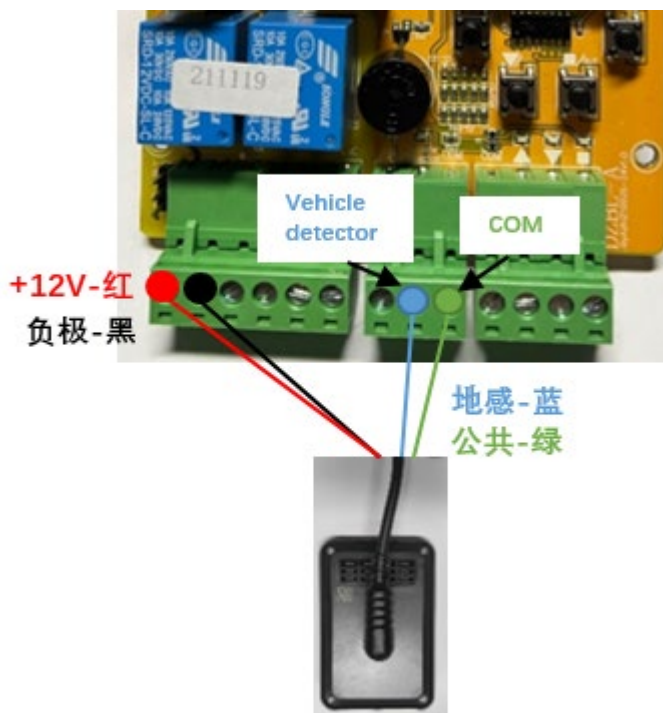
图4-5 防砸雷达电源、信号接线
