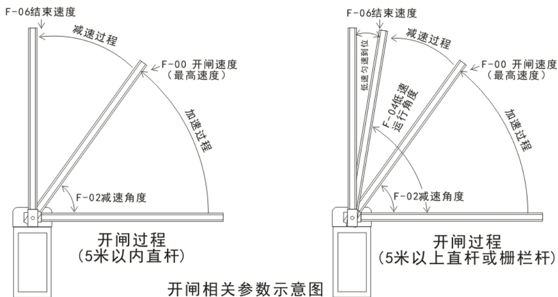
图5-6 开闸相关参数示意图
