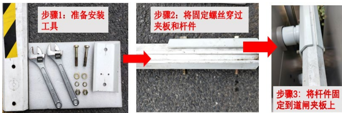
图3-14 伸缩杆闸杆安装图片
