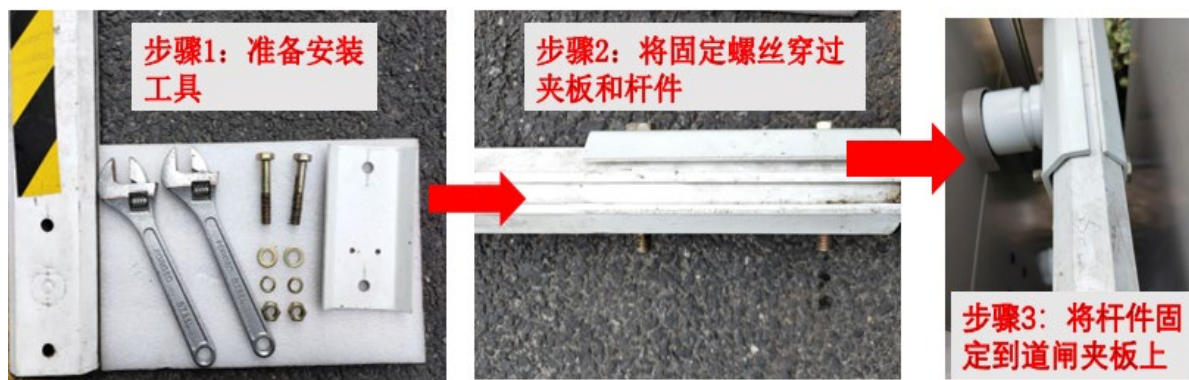
图3-4 直杆带胶条闸杆安装
