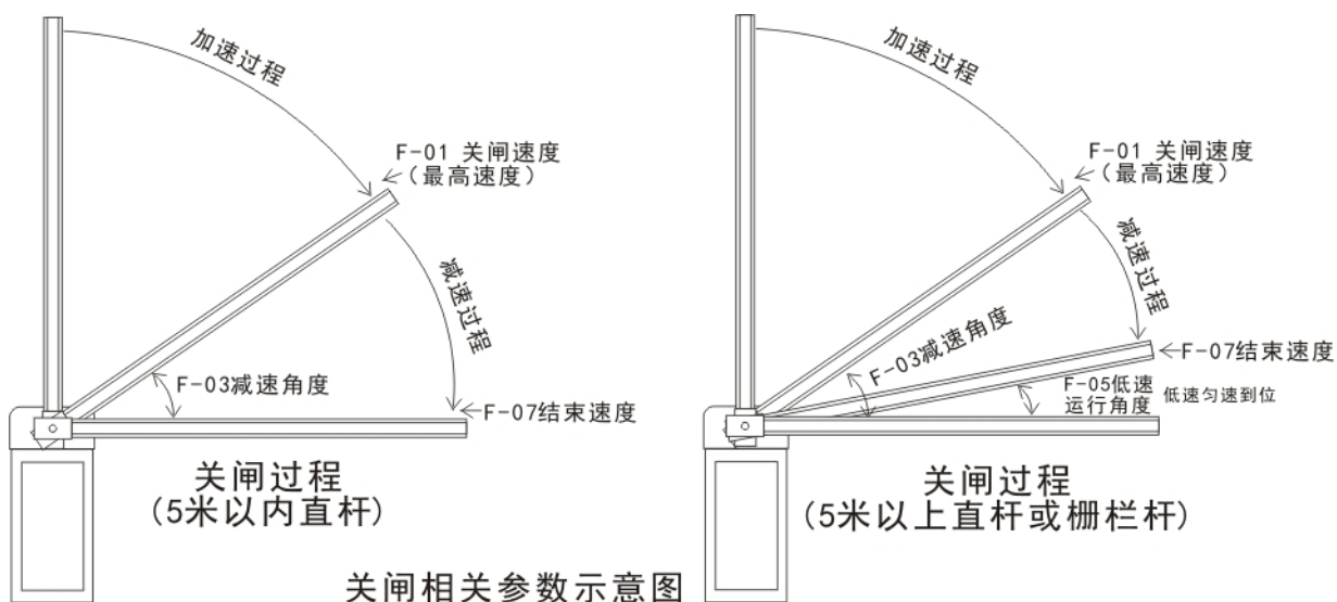
图5-7 关闸相关参数示意图
