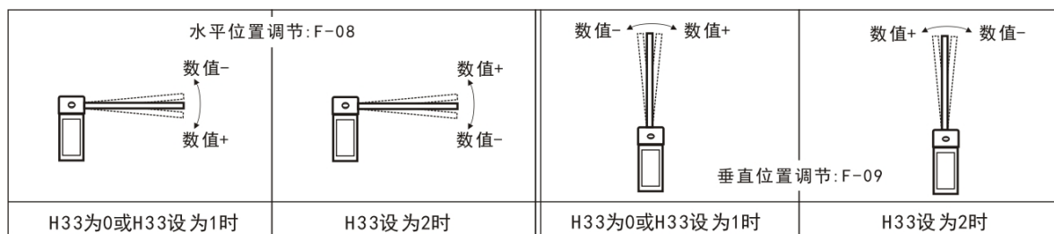
图5-3 F-08 和 F-09 调整说明
