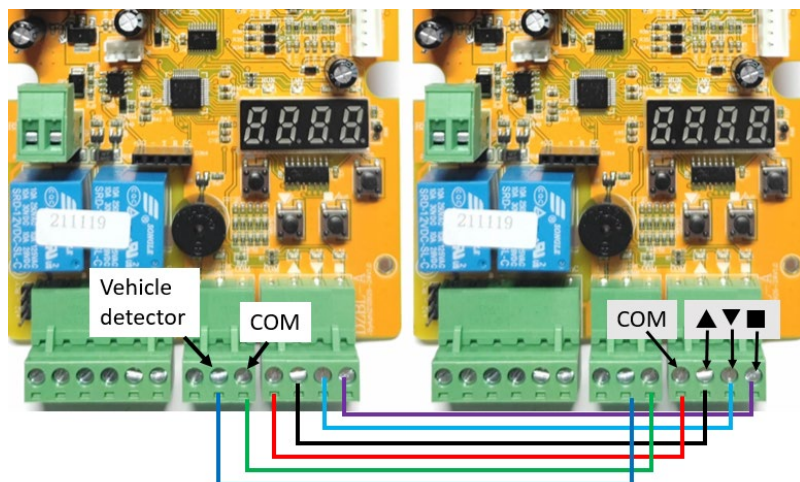
图4-8 对开信号接线
