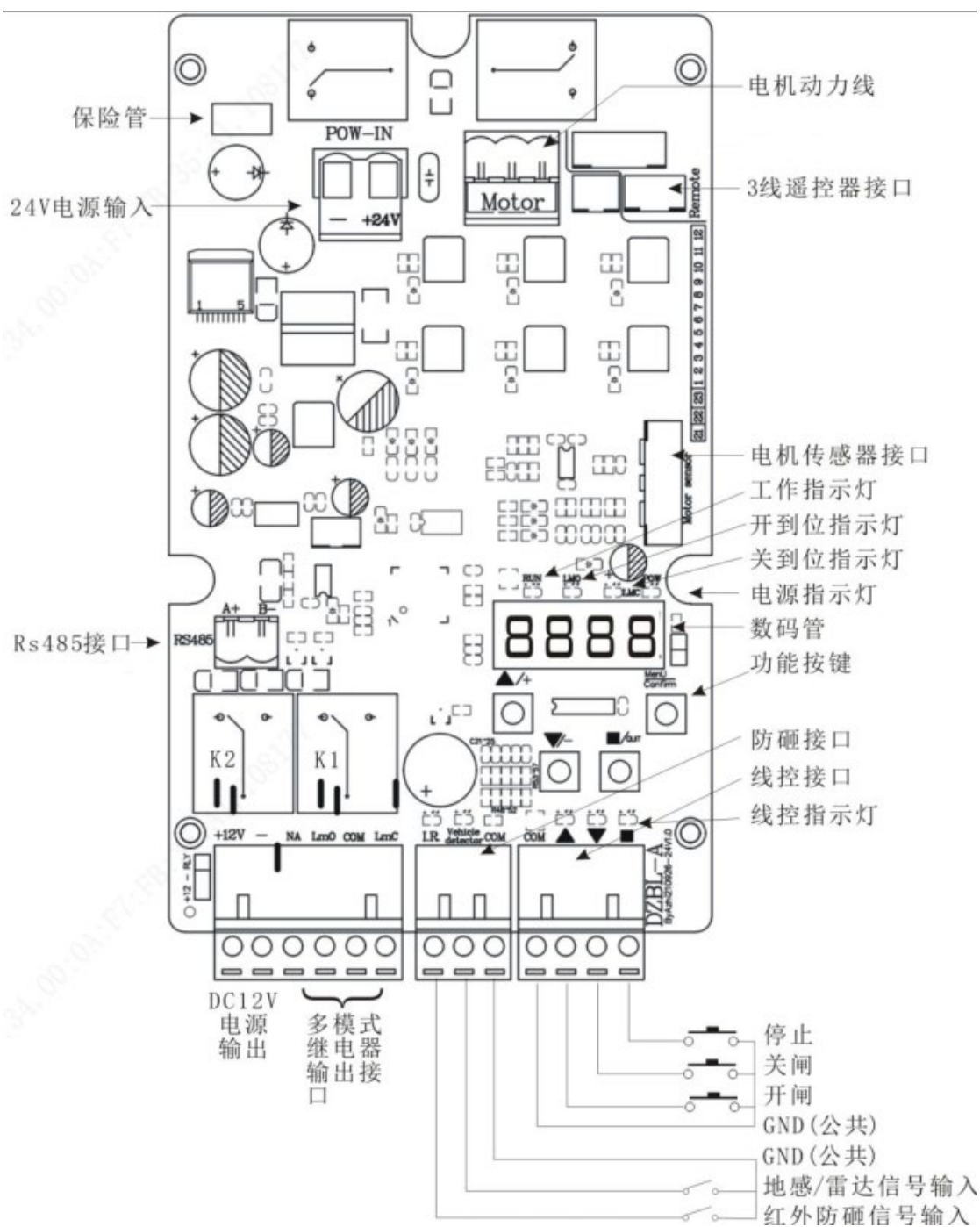
图5-2 控制器示意图
